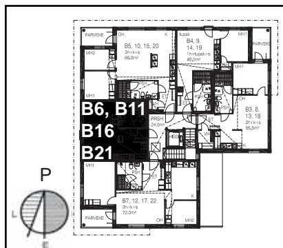
PAIKANNUSKAAVIO 2.-5.krs
